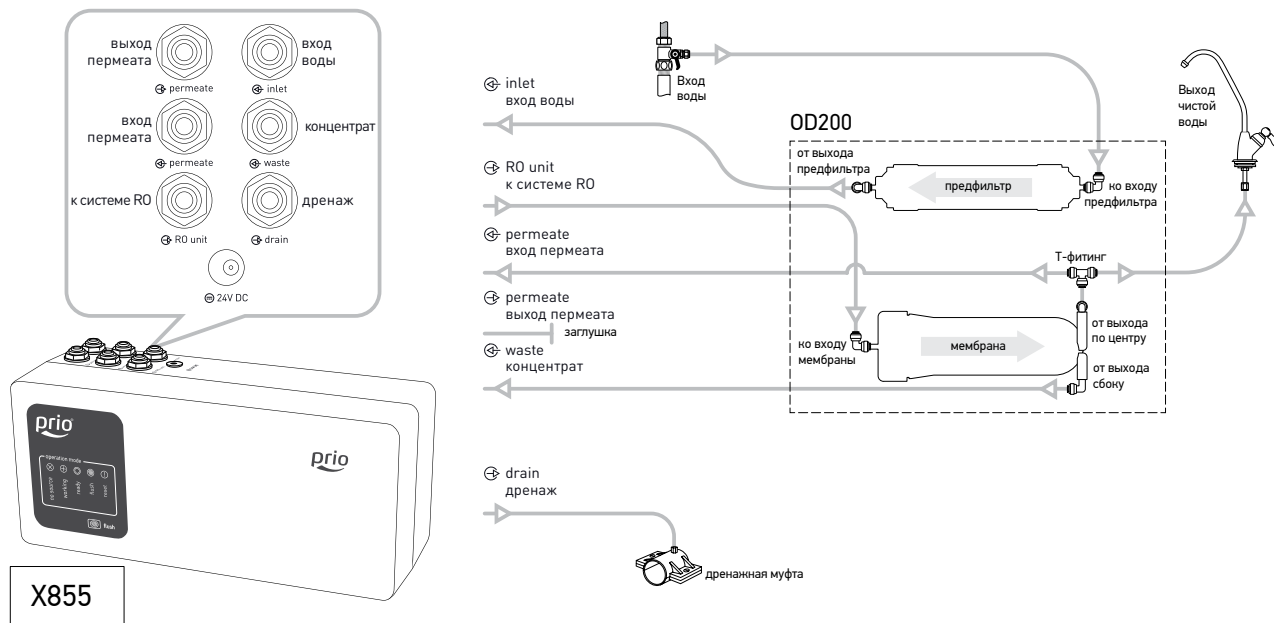
Рис. 11. Добавление помпового блока X855 к проточной системе обратного осмоса Prio® Stream Compact OD200
