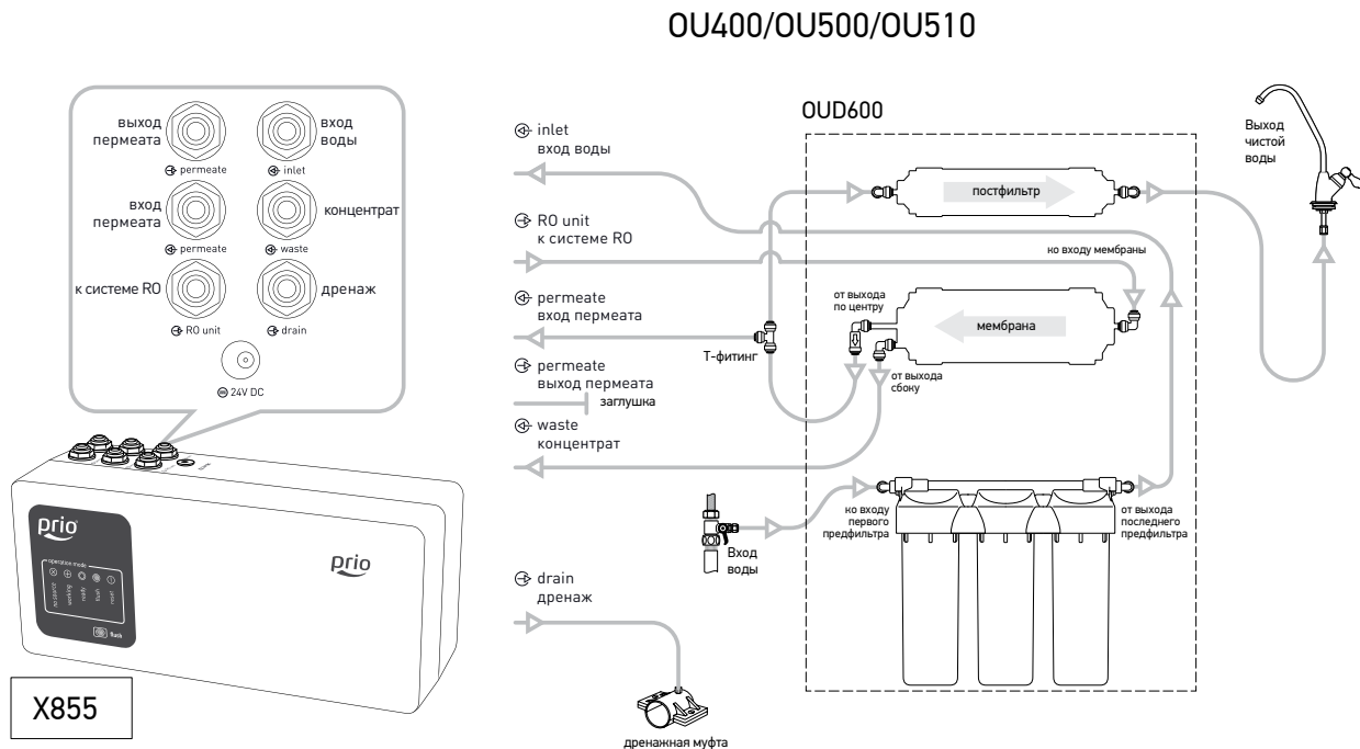
Рис. 13. Преобразование классической системы обратного осмоса с баком и быстросъемной мембраной в проточную систему обратного осмоса с помощью помпового блока X855 (на примере системы Prio® Praktic OU400/OU500/OU510)
