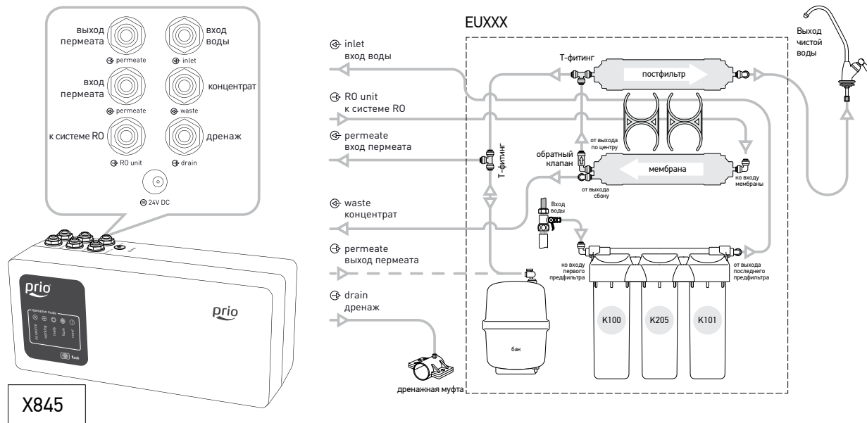
Рис. 15. Преобразование классического многоступенчатого фильтра «под мойку» в систему обратного осмоса с баком и помповым блоком X845 (на примере систем серии Prio® Practic EUXXX)
