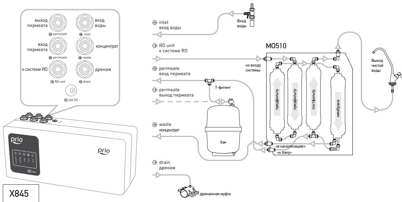
Рис. 9. Добавление помпового блока X845 к системе обратного осмоса Эксперт с баком (на примере системы Prio® Эксперт M0510/M0520/M0530)
