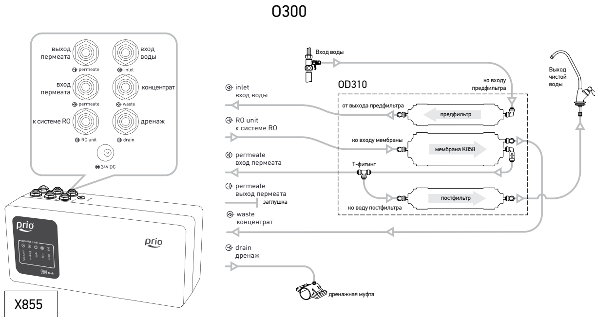
Рис. 14. Преобразование системы обратного осмоса Ecomic с баком в прямоточную систему обратного осмоса с помощью помпового блока X855 (на примере системы Prio® Ecomic O300)
