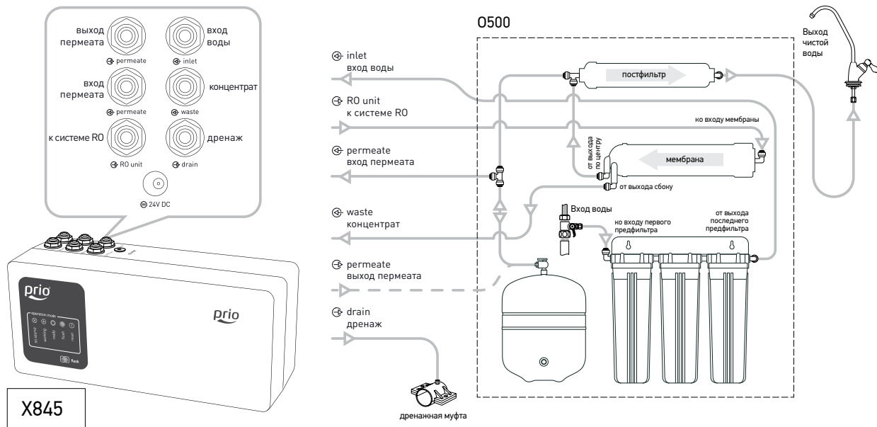
Рис. 7. Добавление помпового блока X845 к классической системе обратного осмоса с баком (на примере системы Новая Вода® O500)
