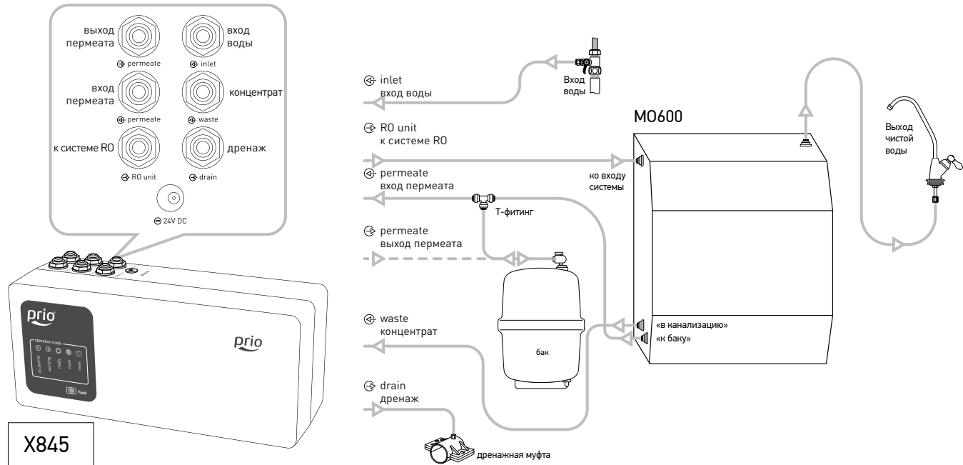
Рис. 4. Схема подключения помпового блока X845 к основному блоку обратноосмотической очистки в составе системы Prio® Expert M0600
