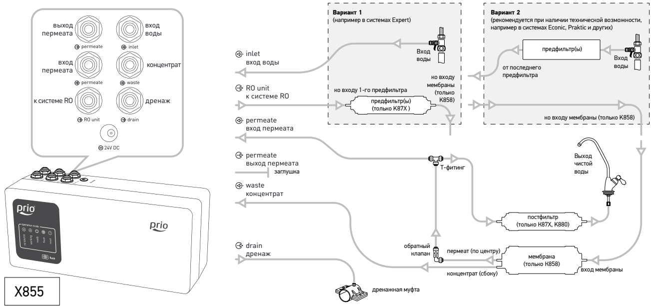
Рис. 2. Принципиальная (функциональная) схема подключения помпового блока X855 к прямоточной системе обратного осмоса
